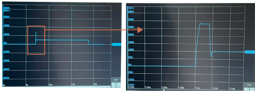
存储记录仪将测试23秒的波形完整记录下来
