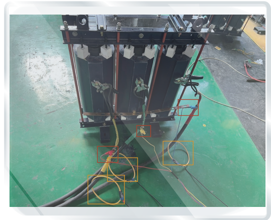
接线方式
